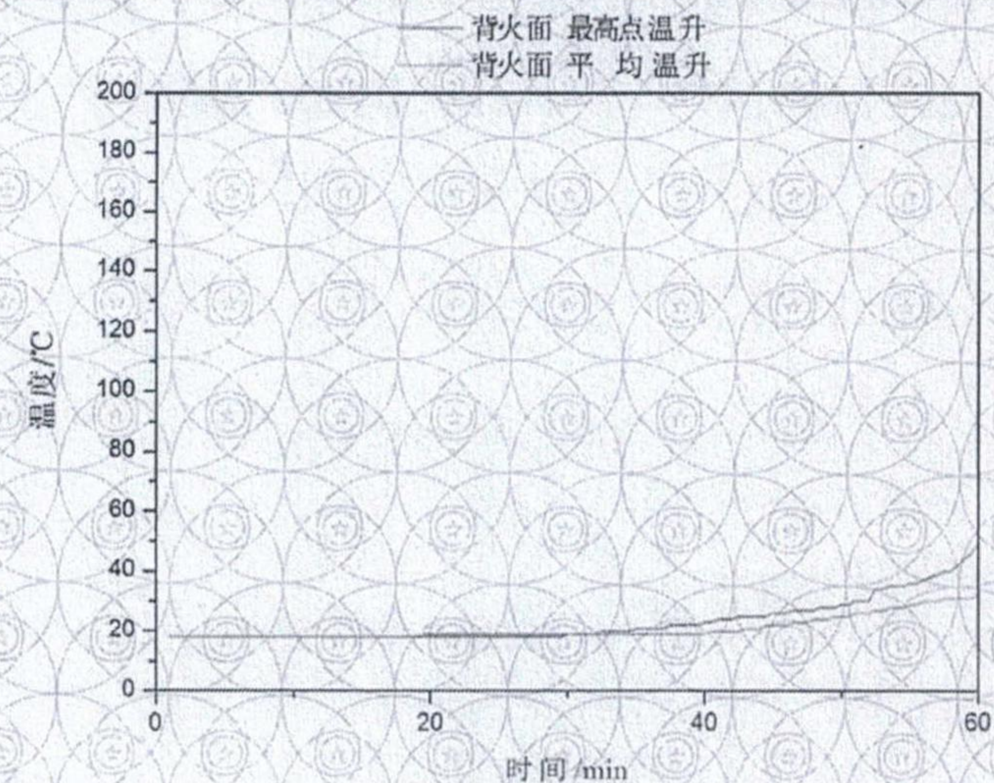
试件背火面温度曲线（背火面按非承重垂直分割构件的要求设置10支热电偶）
