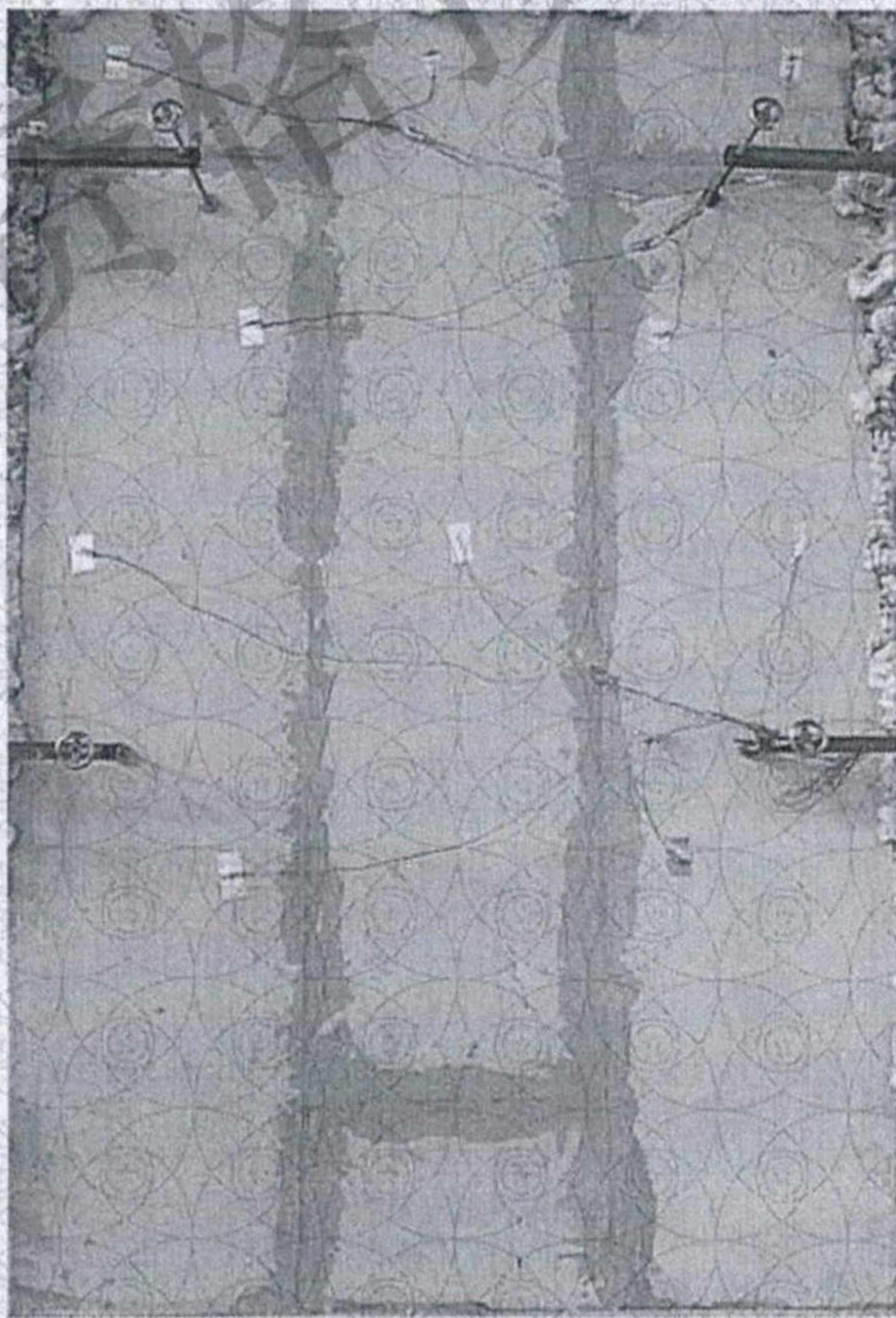
耐火极限试验后照片
